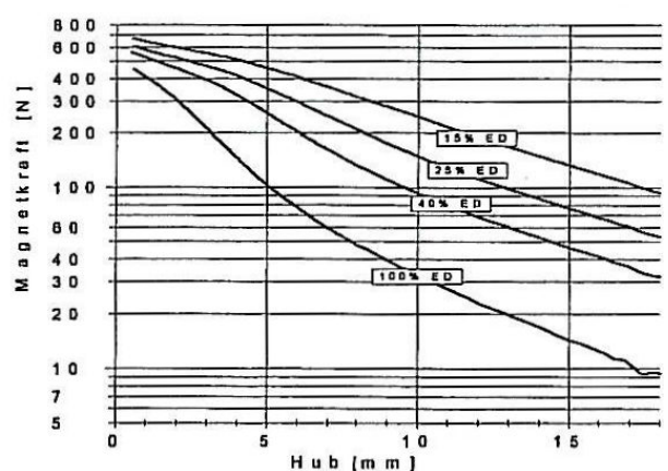
Kraft / Weg-Kennlinie Mit Kühlblech
