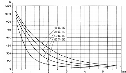
Kraft / Weg-Kennlinie Mit Kühlblech
