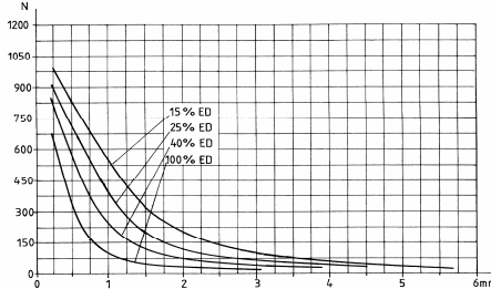
Kraft / Weg-Kennlinie Luftkühlung
